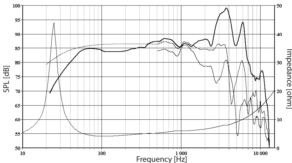
上图所示频率响应曲线是将扬声器单元安装在容积28升的密闭箱上，并在自由场中以轴向0度、离轴30度、60度测试获得的。测试信号2.83伏、麦克风距离0.5米、并将频响曲线标准化至1米测试距离。虚线是该扬声器单元在无限大障板上的频率响应曲线，依据技术数据计算所得。阻抗曲线是在将扬声器单元单独放置在自由场中采用2伏信号测试获得的。
